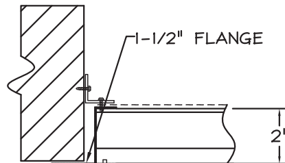
FLANGE FRAME
